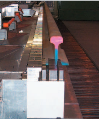
A) Fräsen der Zungen- und Backenschienen auf 2 x 24 m Länge
