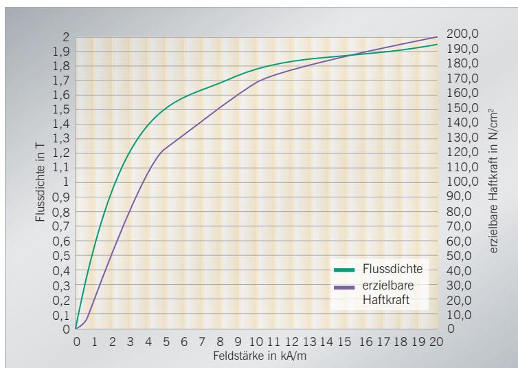
Abb. 2: Magnetisierungskennlinie St37
