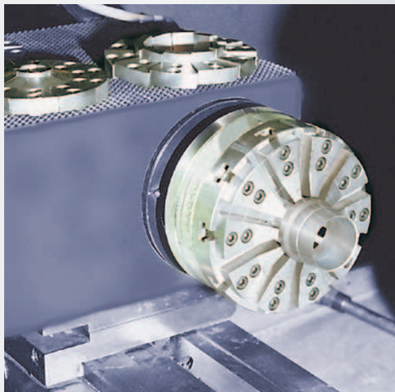
Rundschleifen auf Permanent-Rundmagnet
