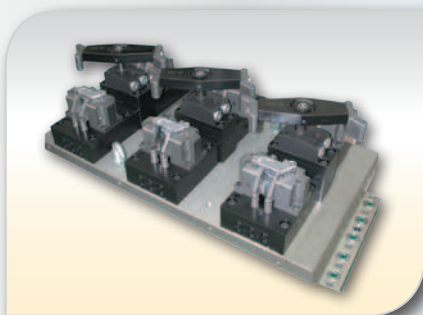
6-fach Spannvorrichtung
