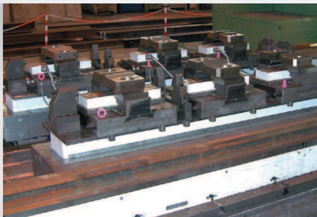
C) Fertigbearbeitung der Herzstücke
