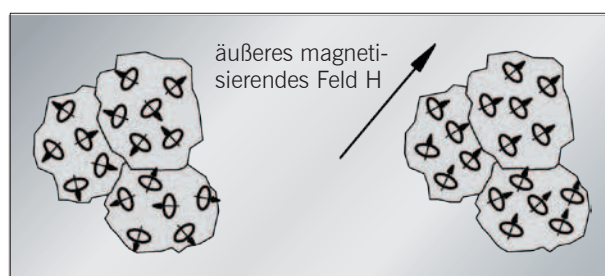
Abb. 6: Ausrichtung der „Molekular-Magnete“ in den Weiß'schen Bezirken durch ein anliegendes Magnetfeld
