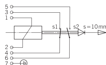
Schaltbild und Kontaktbelegung am Stecker (Magnet stromlos)
