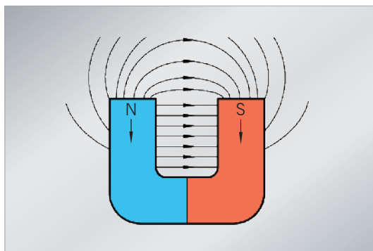
Abb. 4: Veranschaulichung der magnetischen Kraftlinien eines Hufeisenmagnets
